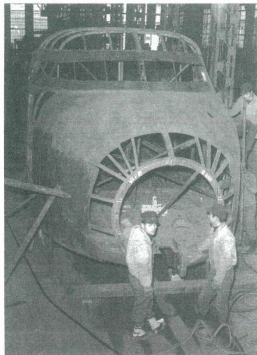
東海道新幹線試作車両
